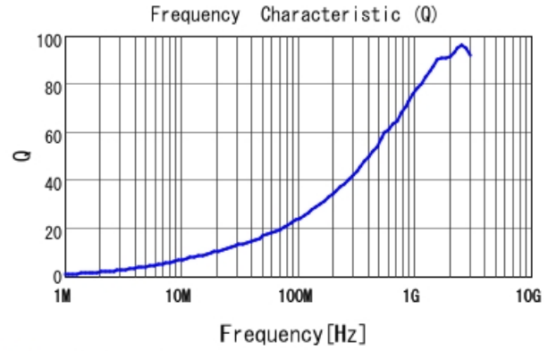
■ LQW15AN6N3G80 Q
