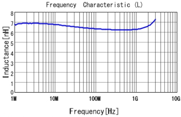
■ LQW15AN6N3G80 L
