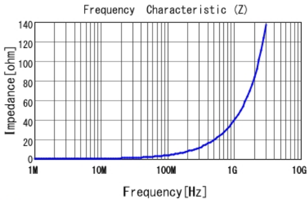
■ LQW15AN6N3G80 |Z|
